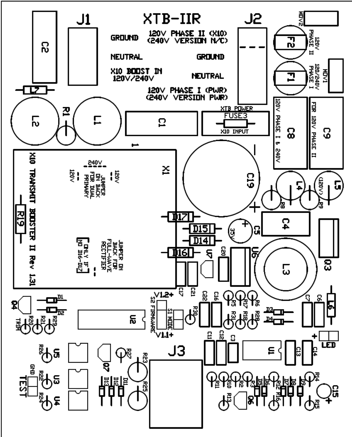
Layer: XTB-II_Rev131.GTO
